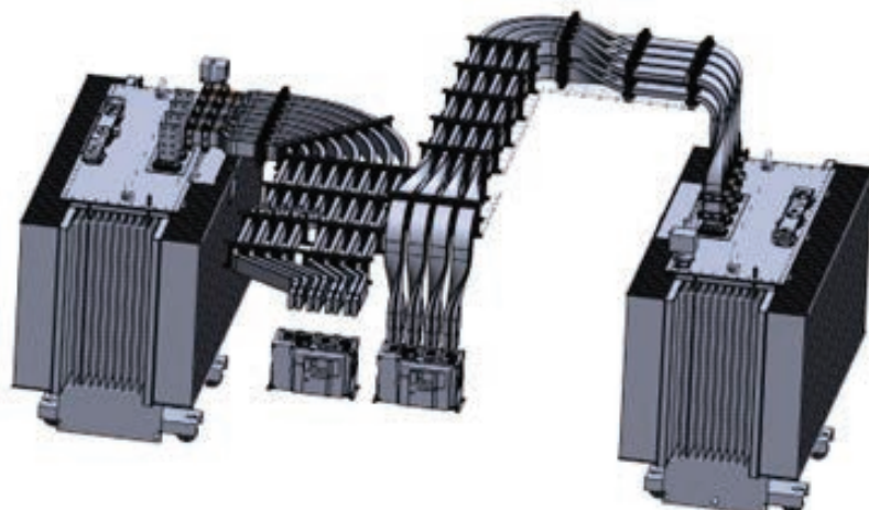
Exemple d'un cheminement Flexbus en 3D
