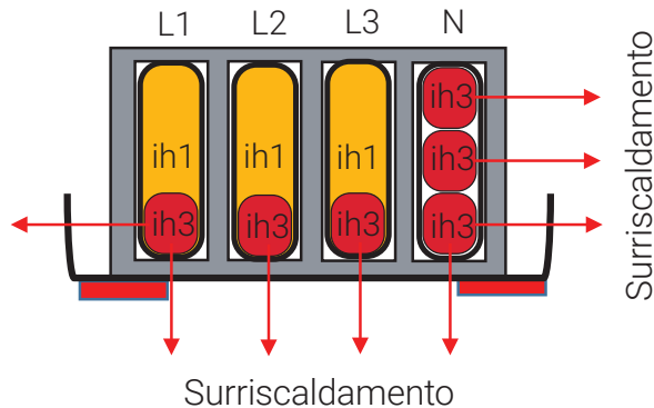
Ih1: Frequenza fondamentale (50 Hz) Ih3: +33% armoniche di ordine 3 (150 Hz)
