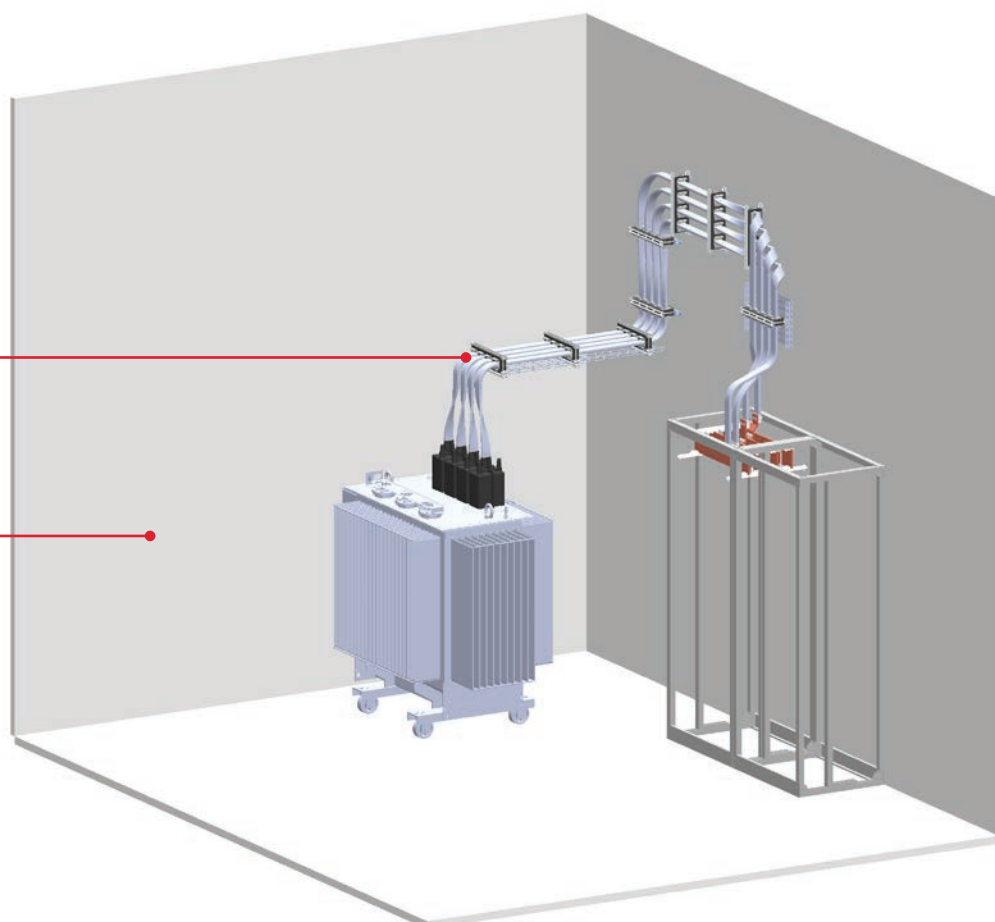
Sala tecnica/Sottostazione/Shelter
