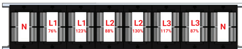
Disposizione dei conduttori non ottimizzata (corrente di carico sbilanciata)
