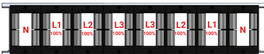
Disposizione ottimizzata del conduttore (corrente di carico bilanciata)
