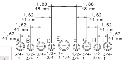
Conduit Sizes
