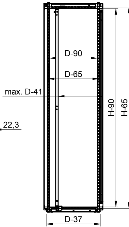
SECTION A-A
