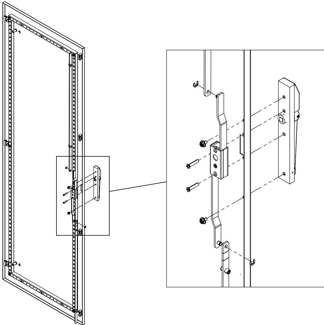
局部视图 A 比例 1 : 4
