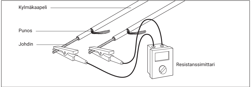
Lämpökaapelin resistanssimittaus
