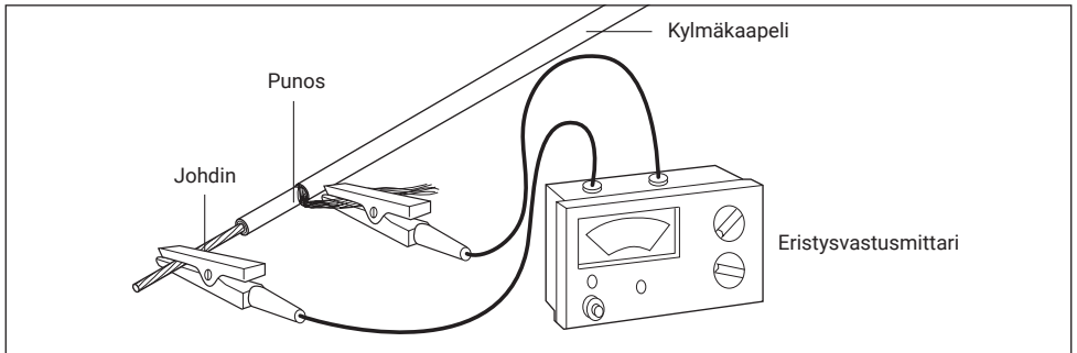
Lämpökaapelin resistanssimittaus
