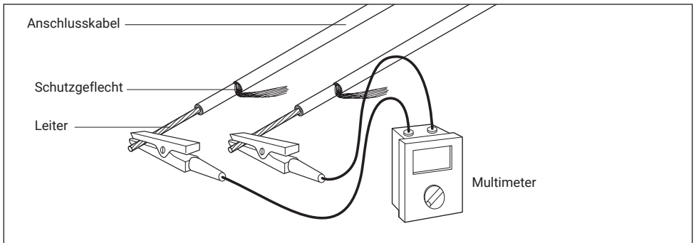
Heizkreiswiderstandsmessung
