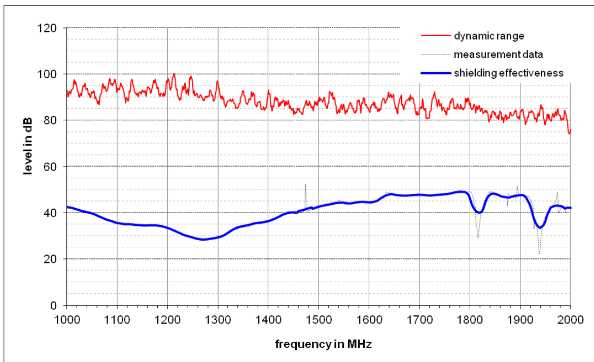
Abbildung 12: Messergebnisse bei direkter Einstrahlung auf die rechte Seitenwand
