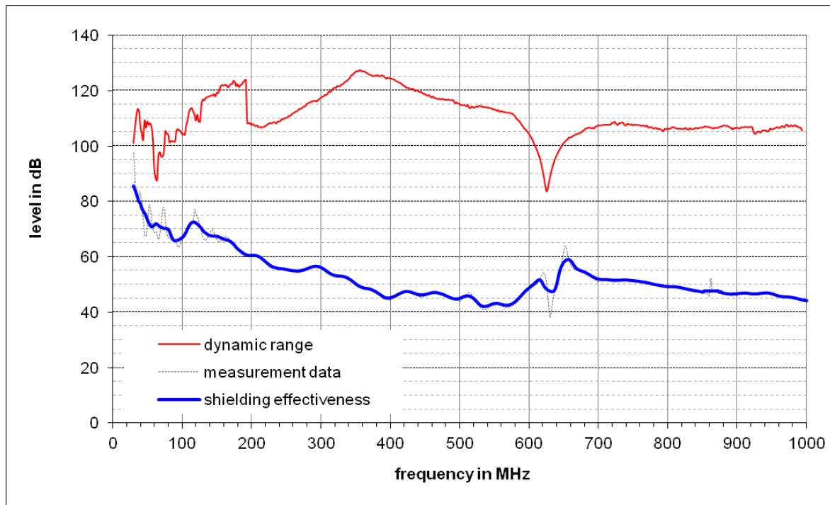
Abbildung 9: Messergebnisse bei direkter Einstrahlung auf die obere Seitenwand
