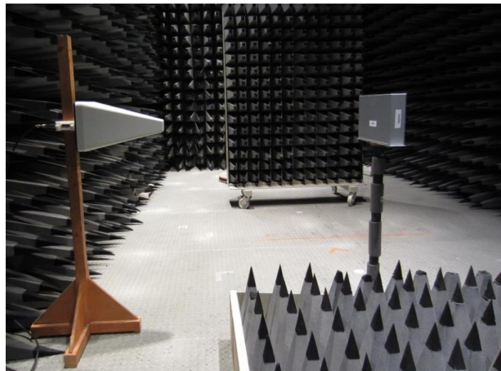
Abbildung 6: Aufbau im Frequenzbereich 1 - 2 GHz
