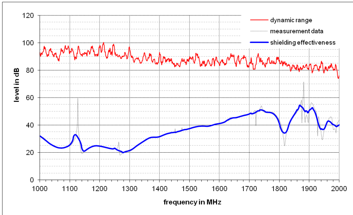
Abbildung 11: Messergebnisse bei direkter Einstrahlung auf die linke Seitenwand
