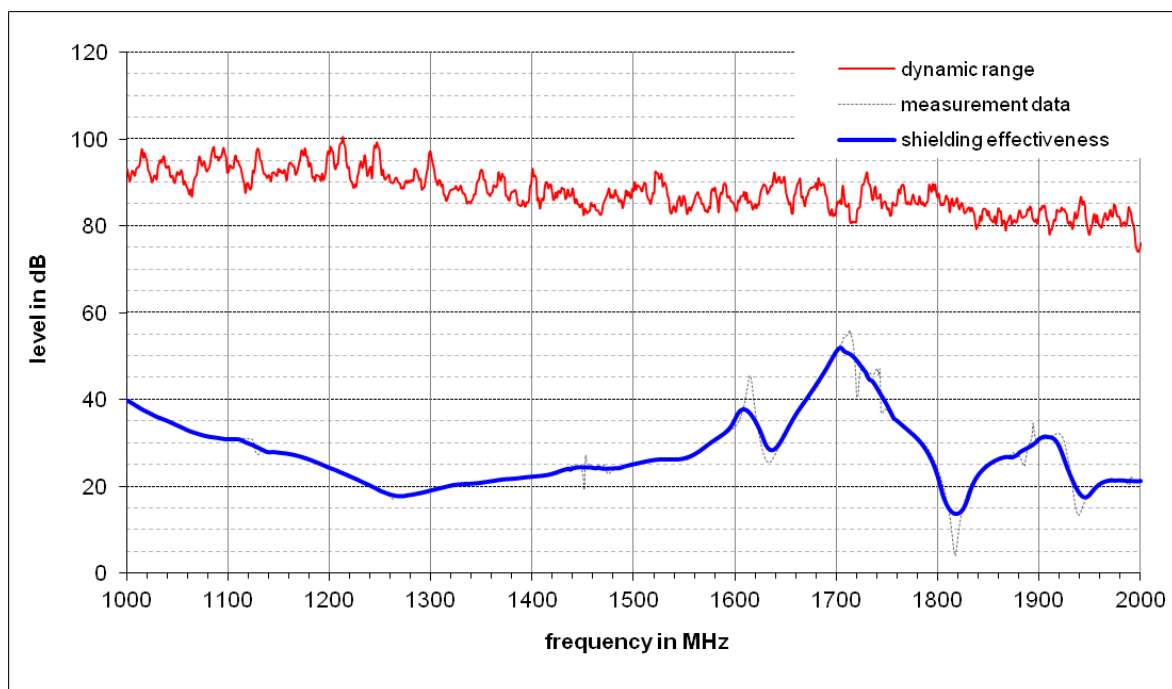
Abbildung 14: Messergebnisse bei direkter Einstrahlung auf die untere Seitenwand
