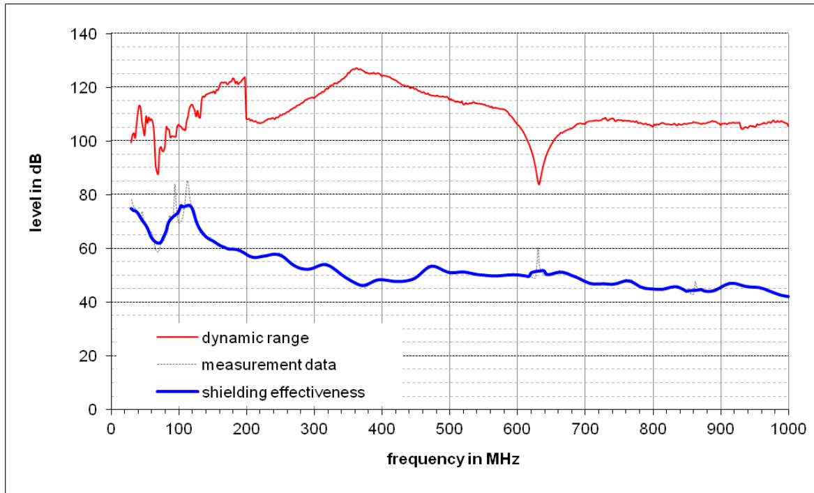
Abbildung 7: Messergebnisse bei direkter Einstrahlung auf die linke Seitenwand
