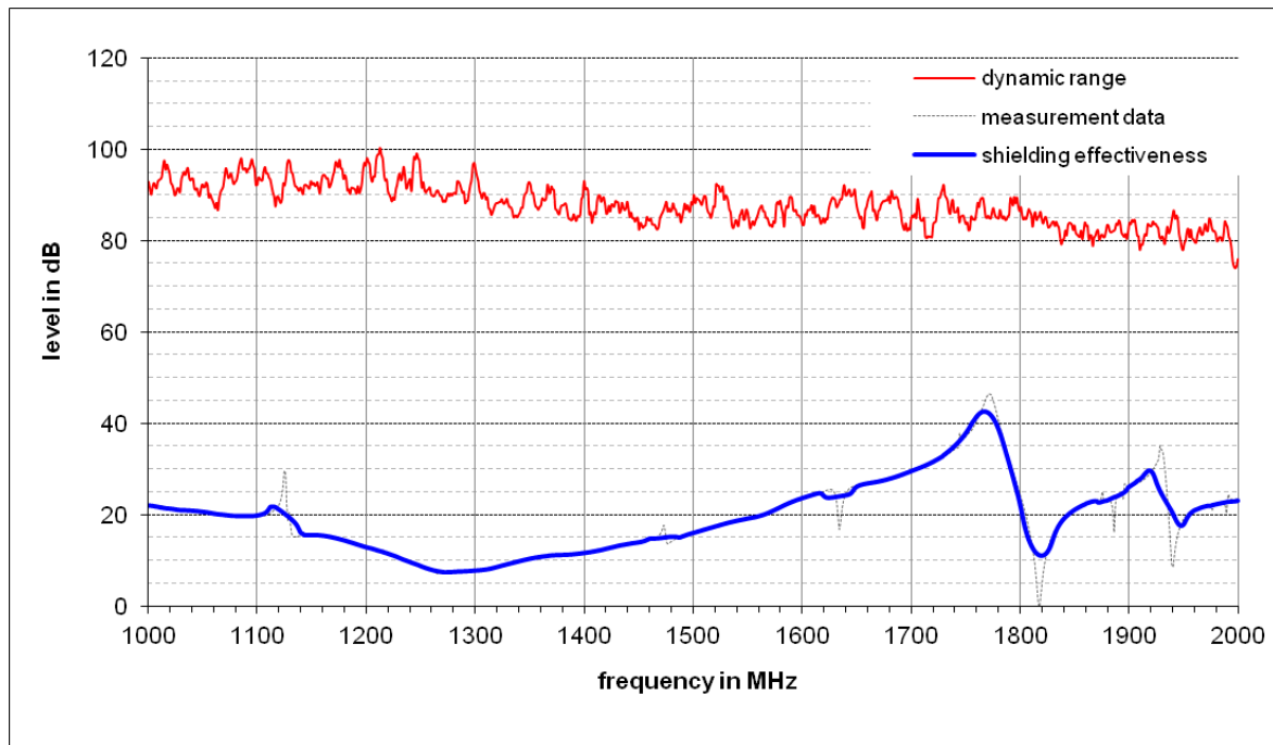
Abbildung 13: Messergebnisse bei direkter Einstrahlung auf die obere Seitenwand
