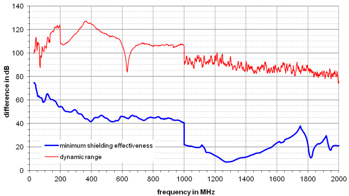
Abbildung 15: Typische Schirmdämpfung und Worst-Case-Abschätzung des Prüfobjekts
