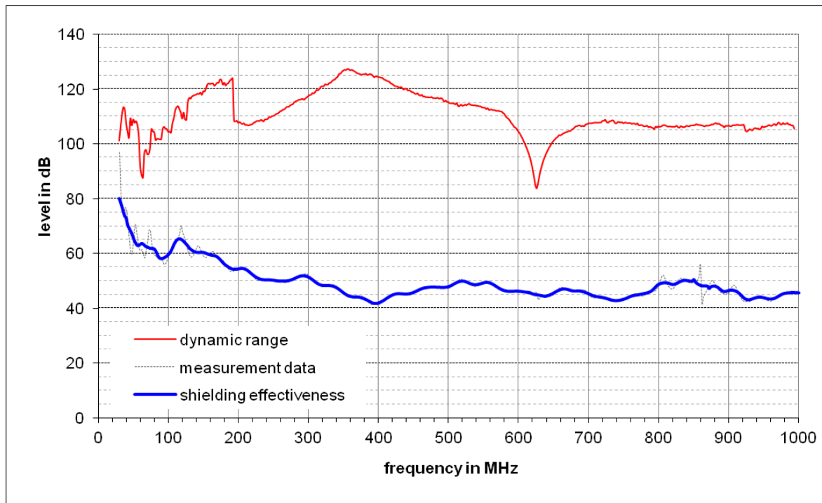
Abbildung 10: Messergebnisse bei direkter Einstrahlung auf die untere Seitenwand
