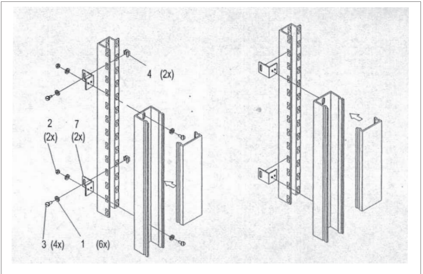
Kabelkanal
