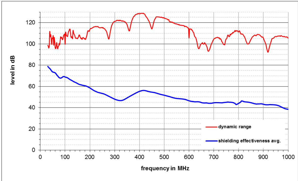
Abbildung 9: Mittelwert der Schirmdämpfungen von G1, G2, G3 bei direkter Einstrahlung auf die obere Seitenwand
