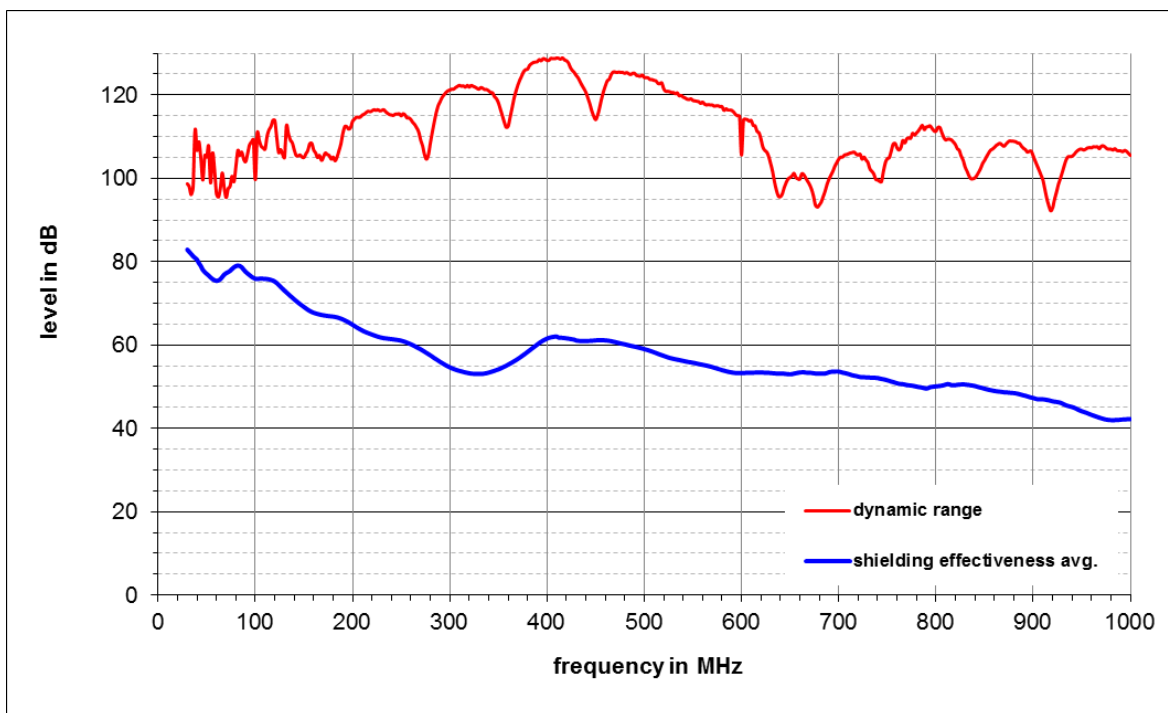
Abbildung 8: Mittelwert der Schirmdämpfungen von G1, G2, G3 bei direkter Einstrahlung auf die rechte Seitenwand
