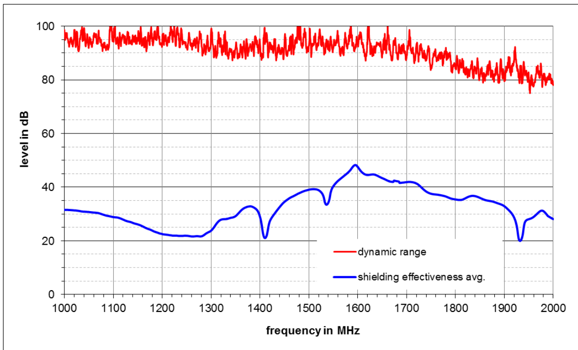
Abbildung 14: Mittelwert der Schirmdämpfungen von G1, G2, G3 bei direkter Einstrahlung auf die untere Seitenwand
