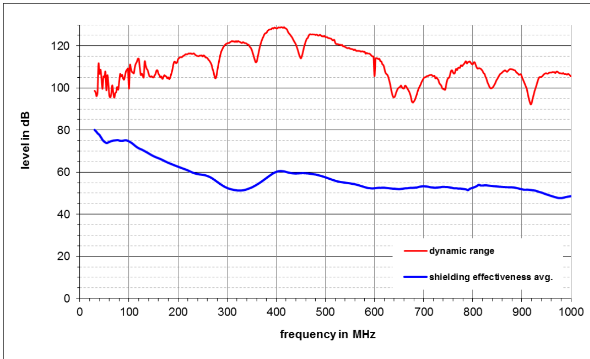
Abbildung 7: Mittelwert der Schirmdämpfungen von G1, G2, G3 bei direkter Einstrahlung auf die linke Seitenwand
