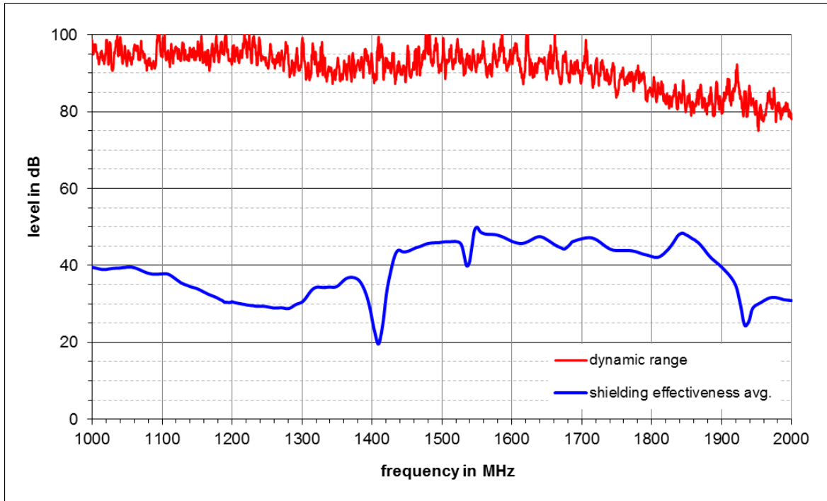
Abbildung 13: Mittelwert der Schirmdämpfungen von G1, G2, G3 bei direkter Einstrahlung auf die obere Seitenwand
