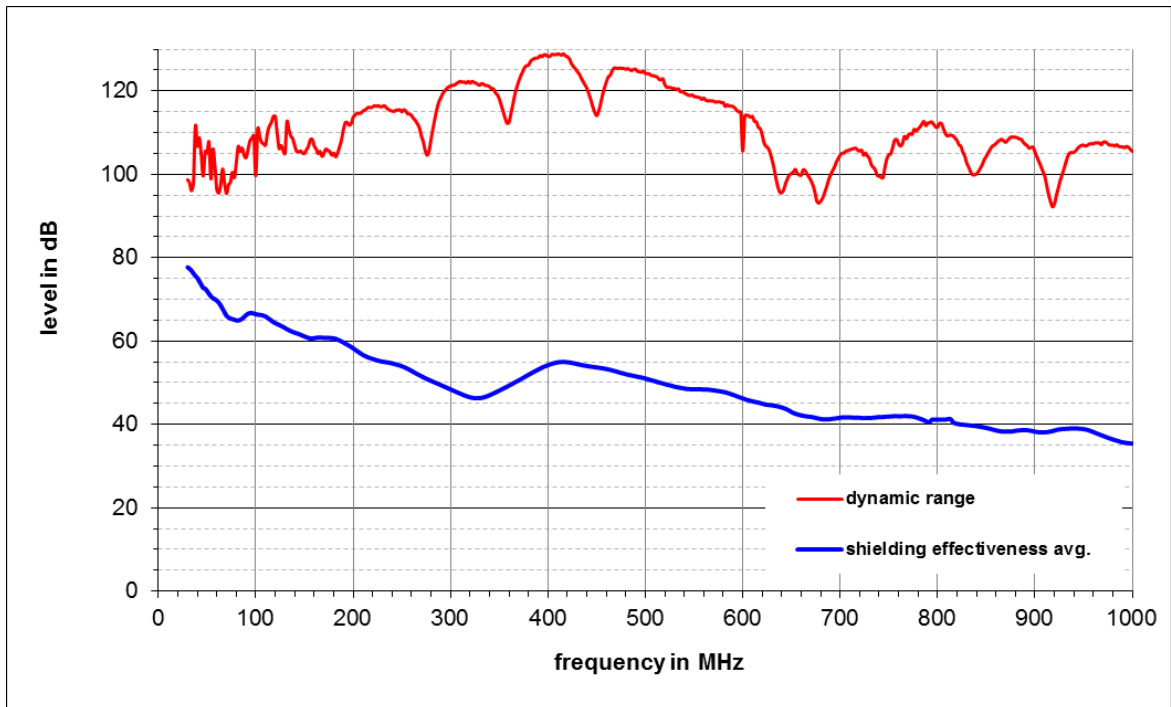
Abbildung 10: Mittelwert der Schirmdämpfungen von G1, G2, G3 bei direkter Einstrahlung auf die untere Seitenwand
