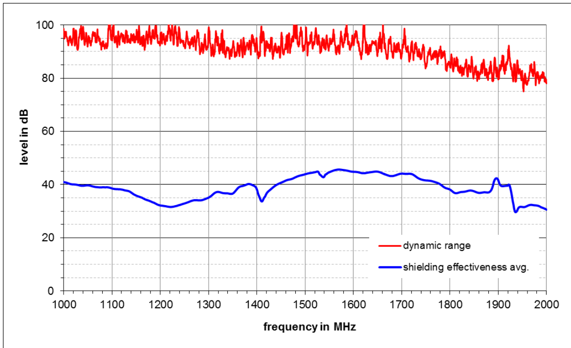
Abbildung 11: Mittelwert der Schirmdämpfungen von G1, G2, G3 bei direkter Einstrahlung auf die linke Seitenwand
