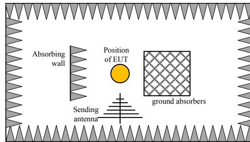
Abbildung 2: Aufbau 1 GHz – 2 GHz
