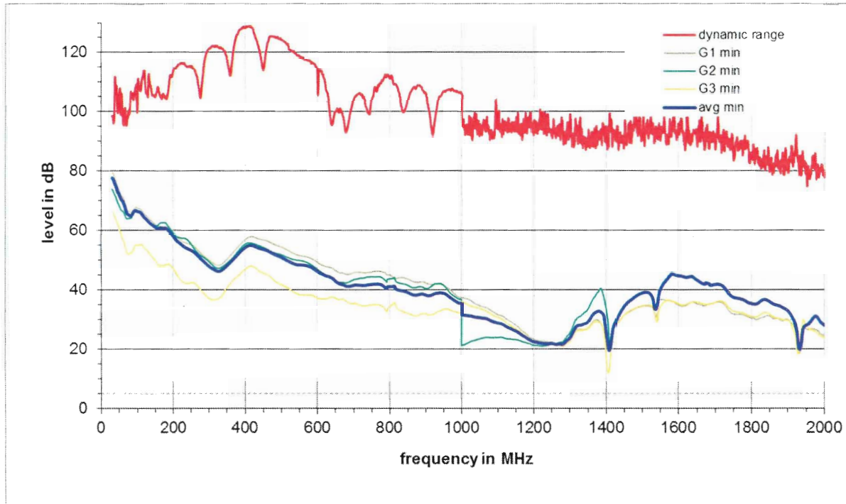
Abbildung 15: Typische Schirmdämpfung und Worst-Case-Abschätzung für Gehäuse 1, 2, 3 und den Mittelwert
