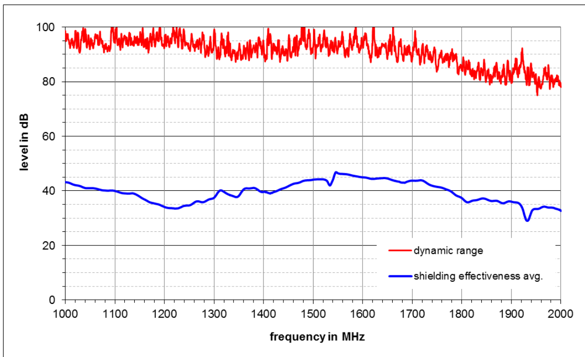
Abbildung 12: Mittelwert der Schirmdämpfungen von G1, G2, G3 bei direkter Einstrahlung auf die rechte Seitenwand
