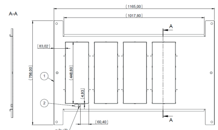
Toit pour passage de câbles
