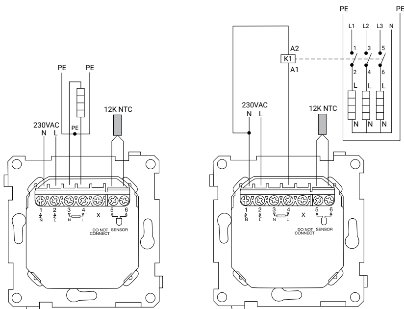
K1: kontaktor med integrert demping
