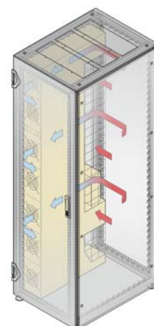
Sechs leistungsstarke, temperaturgeregelte Ventilatoren. Einfacher Zugriff zu Wartungszwecken bei laufendem Betrieb
