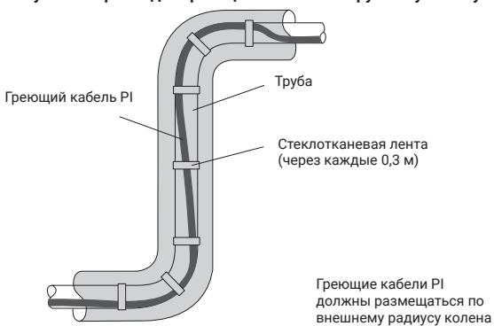
Рисунок 9: Прокладка греющего кабеля по трубному колену
