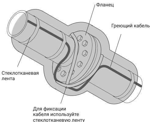
Рисунок 10: Размещение греющего кабеля на фланце
