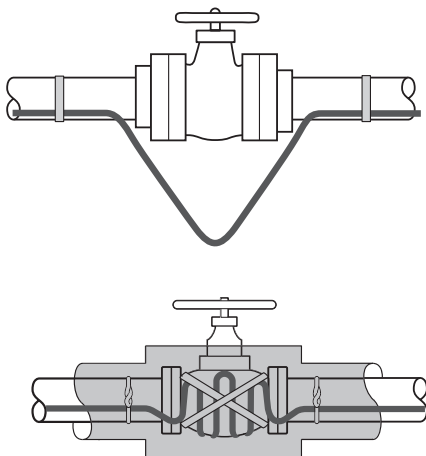
Рисунок 8: Размещение запаса греющего кабеля на клапане
