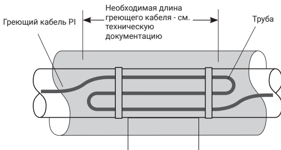
Рисунок 7: Размещение запаса греющего кабеля на трубном башмаке
