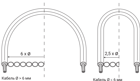
Рисунок 13: Минимальный радиус изгиба греющего кабеля
