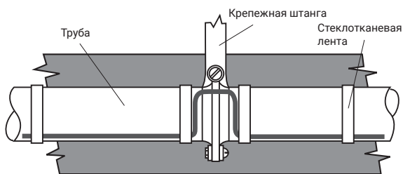
Рисунок 15: Прокладка греющего кабеля над хомутами и зажимами
