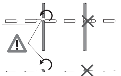
Рисунок 6: Элемент фиксации – перфорированный стальной хомут
