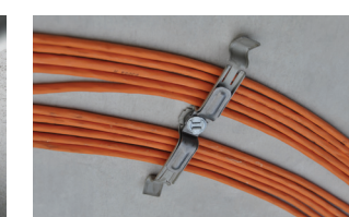
Kabels vanaf/aan betonnen plafond/wand
