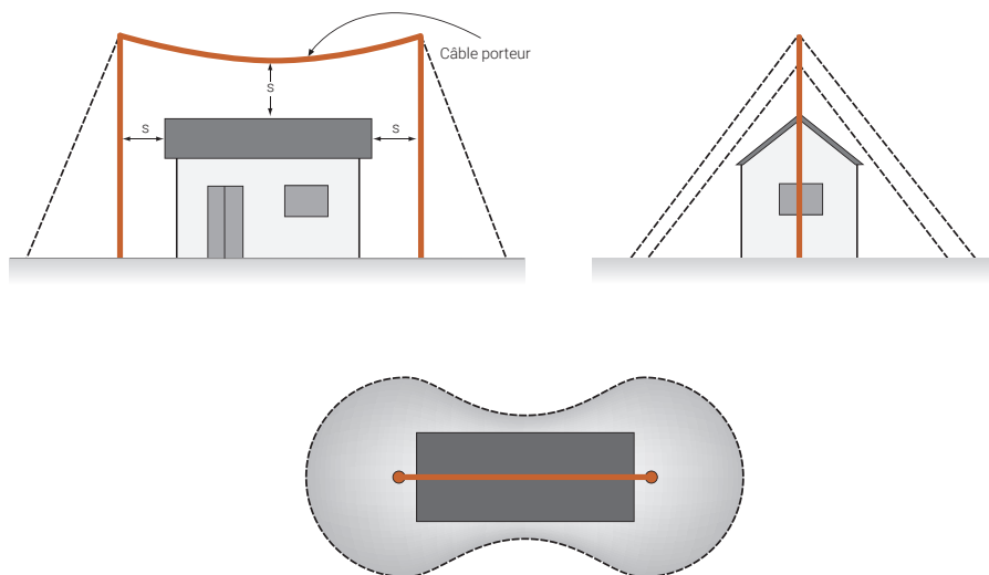
Figure 2 : Méthode de l'angle de protection
