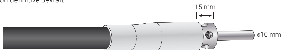
Figure 53 : Terminaison basse terminée
