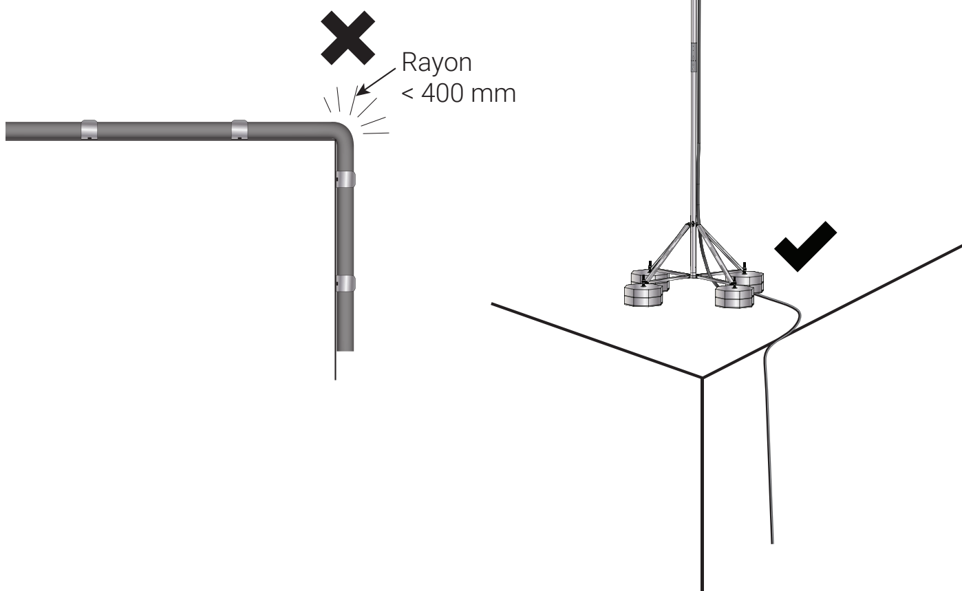
Figure 51 : Exigences de maintien d'un rayon de courbure minimum
