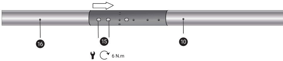
Figure 19 : Assemblage des pièces supérieure et inférieure du mât
