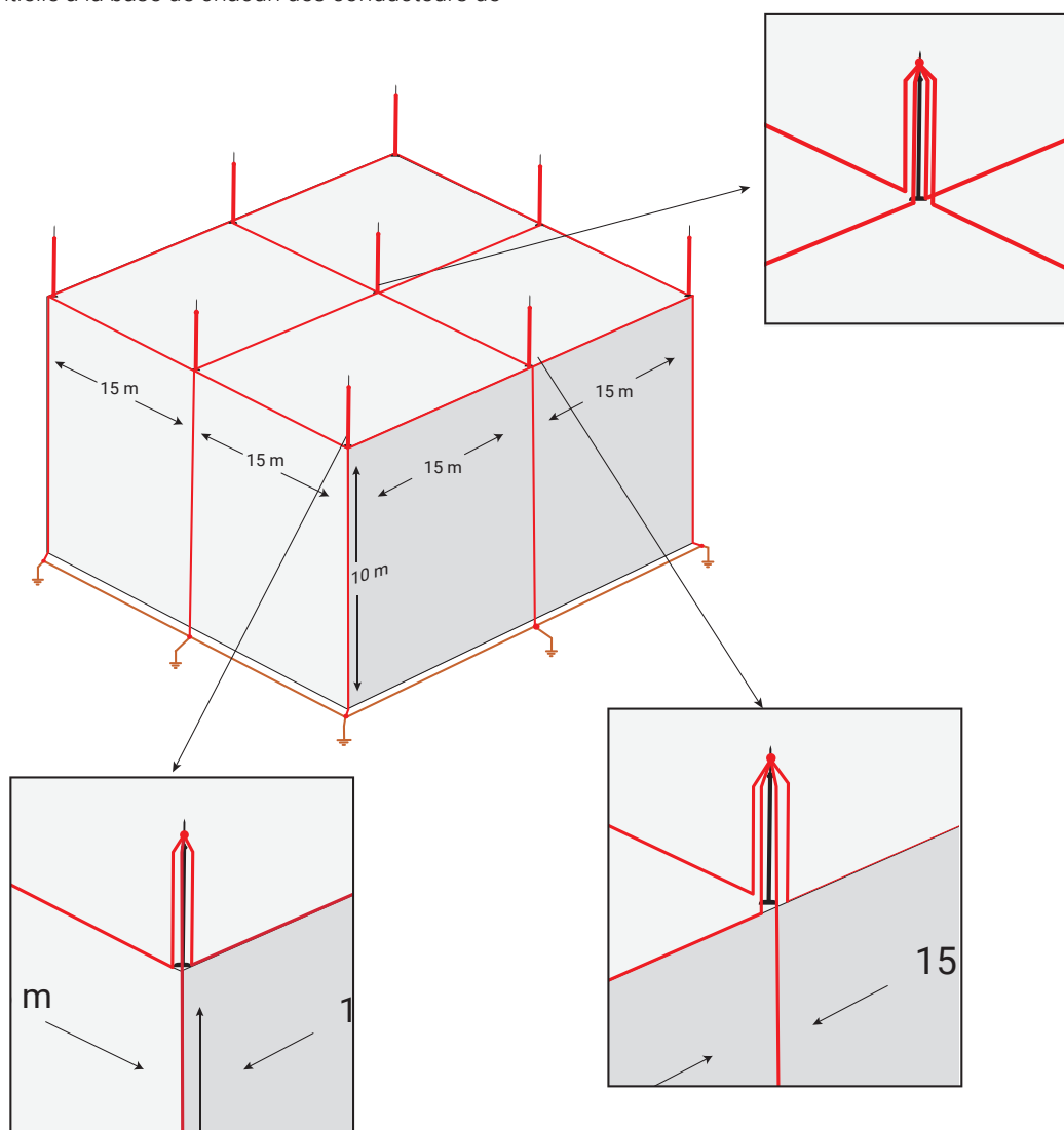
Figure 7 : Couverture complète du bâtiment
