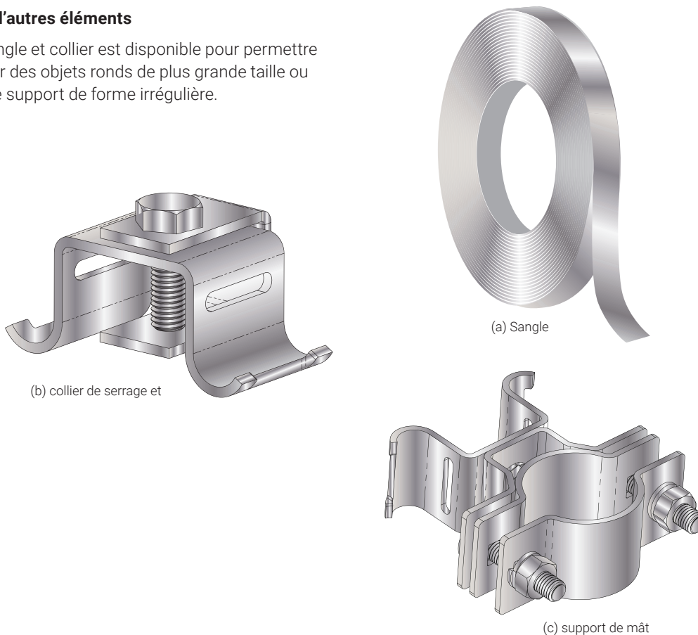
Figure 42 : (a) Sangle, (b) collier de serrage et (c) support de mât
