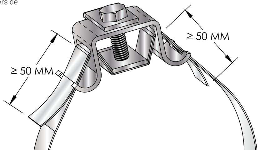
Figure 44 : Dépassement des extrémités de la sangle dans le collier de serrage
