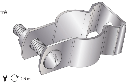
Figure 49 : Élément de fixation ISO n VFS
