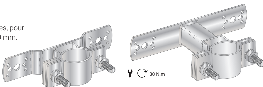
Figure 39 : Supports muraux de petite taille
