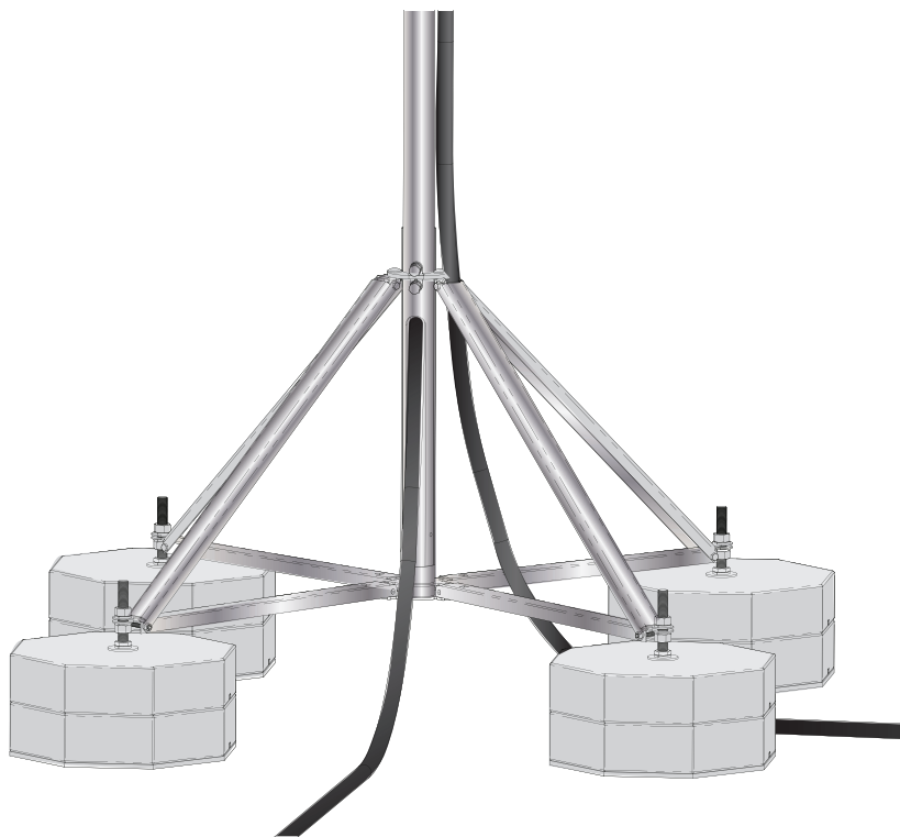
Figure 32 : Disposition de blocs de béton sur une surface horizontale
