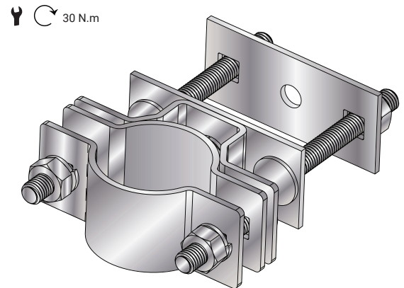
Figure 45 : Raccord d'installation sur un profilé rectangulaire ou carré
