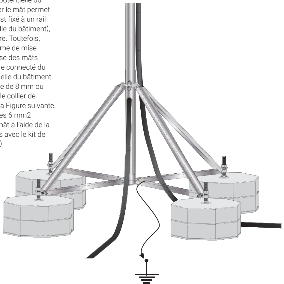
Figure 46 : Connexion du conducteur de liaison
