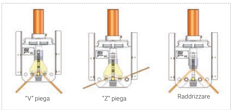
PIEGABARRE IDRAULICA PER BARRE IN RAME
